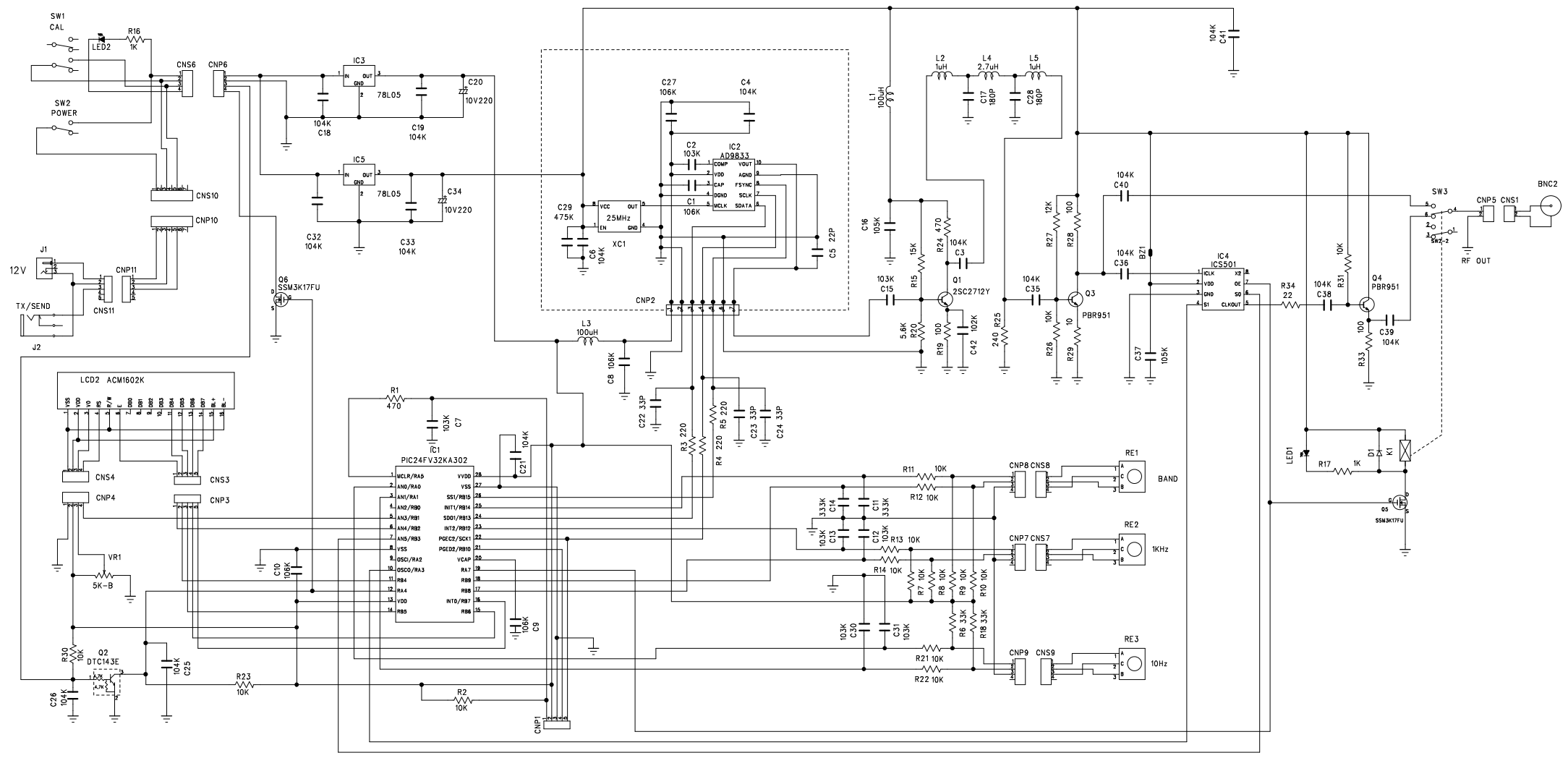
AD9833 DDS (1-50MHz VFO)
