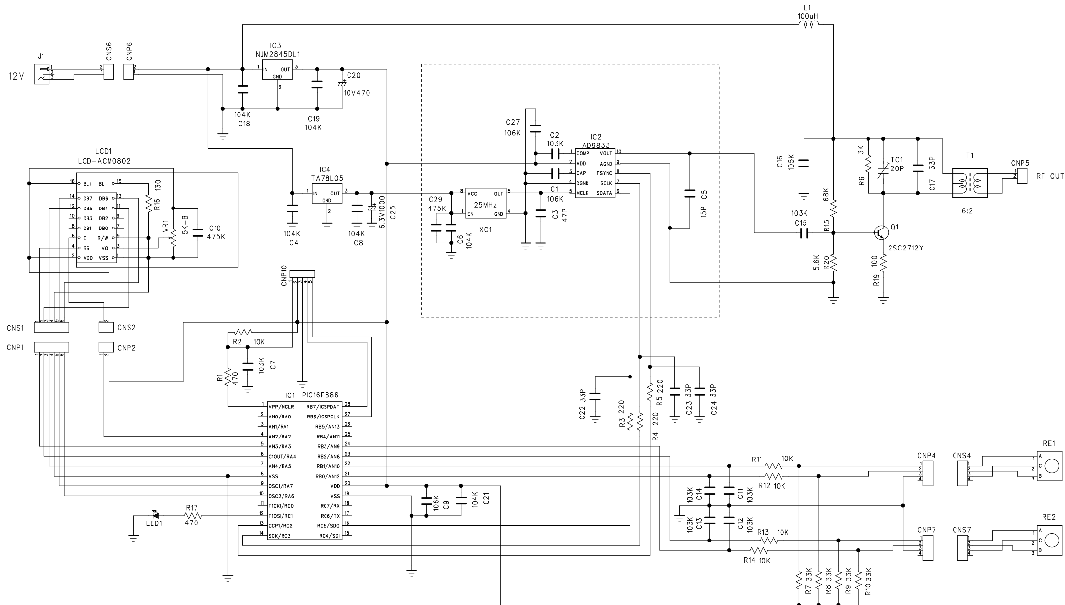
AD9833 DDS (7MHz VF0)
