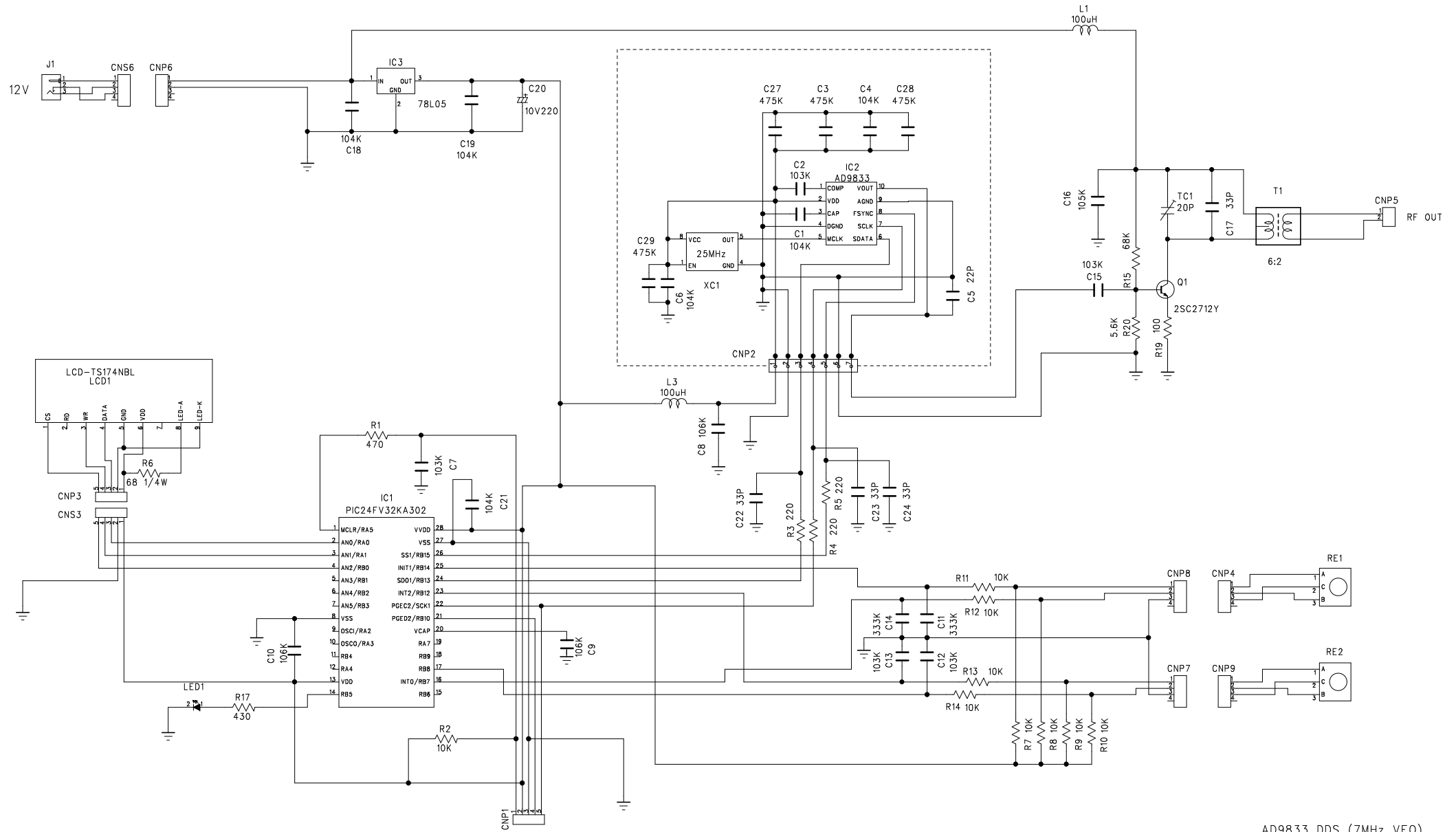
AD9833 DDS (7MHz VFO)
