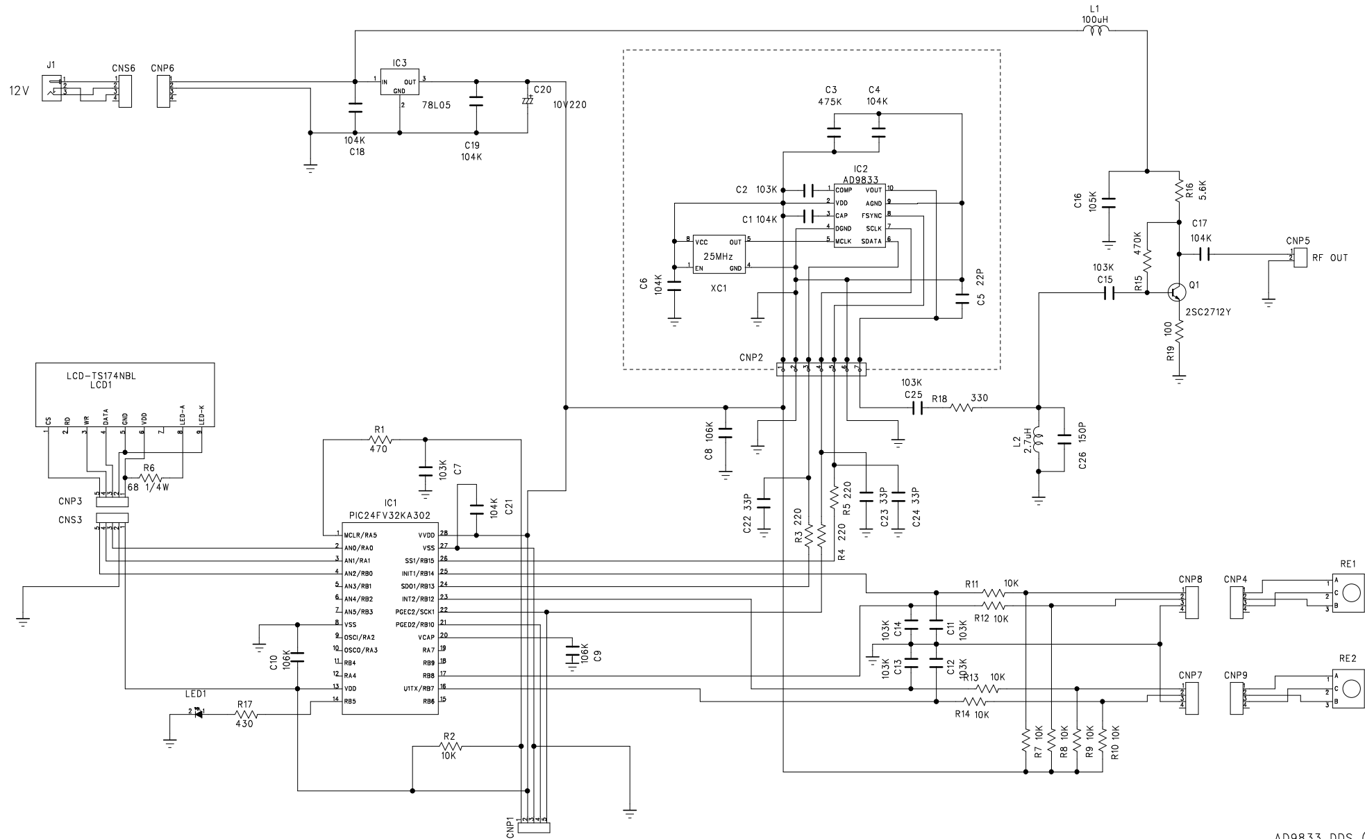
AD9833 DDS (7MHz VFO)
